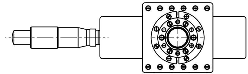
Rückansicht Maßstab: 1:2
